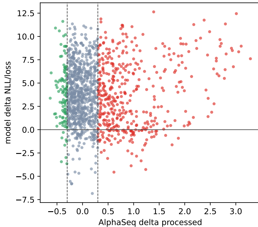
AbLang2
