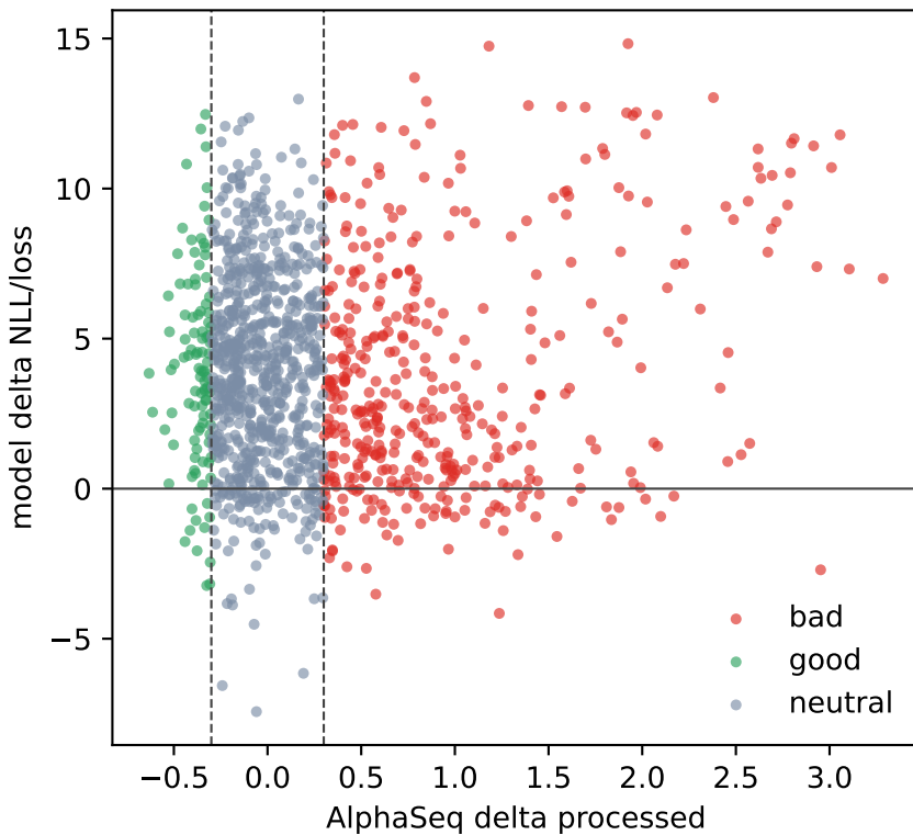
ESM2
